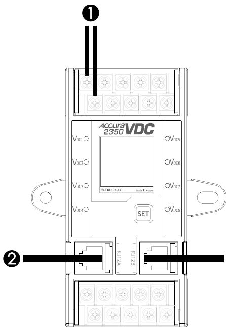
Fig 1.7 DC 전압 및 통신선 결선
