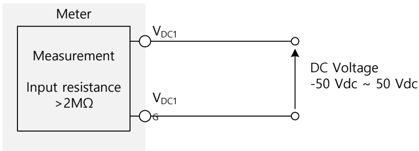
Fig 2.2 아날로그 입력 DC 전압
