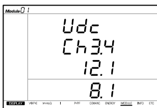
Fig 3.2 채널 3,4 DC 전압 표시 화면
